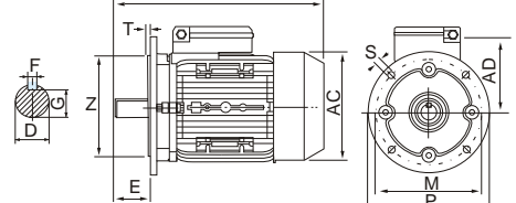
IMB5
