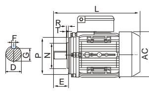
IMB14
