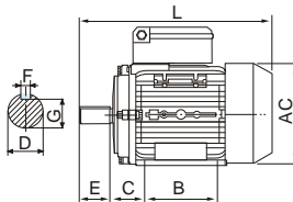
IMB3
